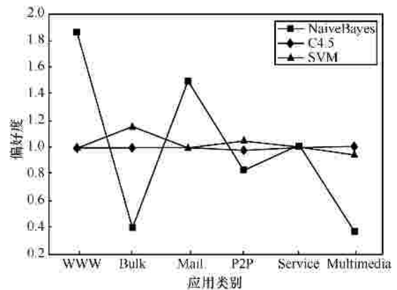
图 2 不同分类器对不同类别的偏好度
