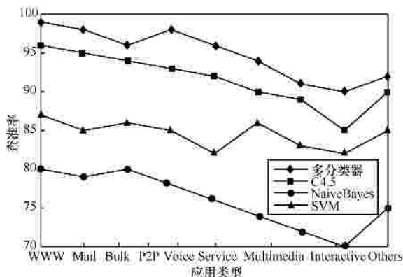
图 4 多分类器与传统机器学习算法查准率
