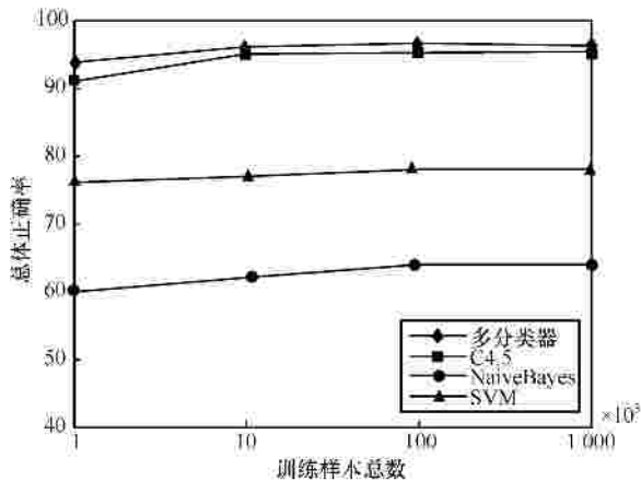
图 6 样本大小对识别正确率的影响
