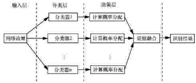
图 1 多分类器融合流量识别模型
